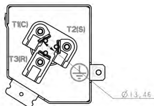
壓縮機接線示意圖
